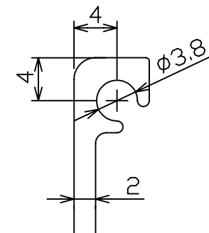
A部詳細 (2:1)
