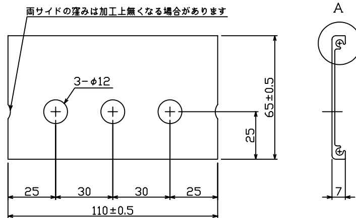
TYPE : UPS-A3
